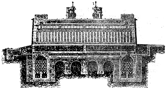
Фиг. 4. Печь Отто-Гофманна.
