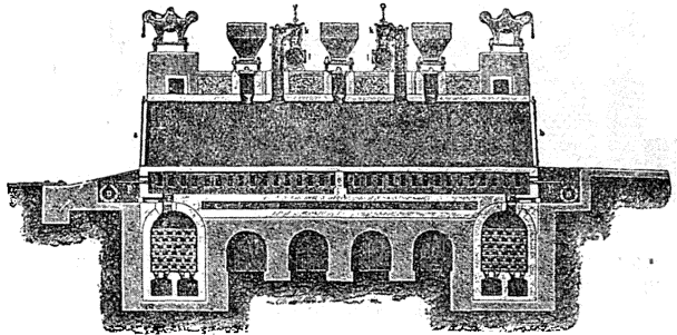
Фиг. 3. Печь Отто-Гофманна.
