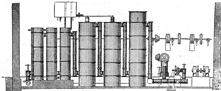
Фиг. 8. Конденсационный приборъ.
