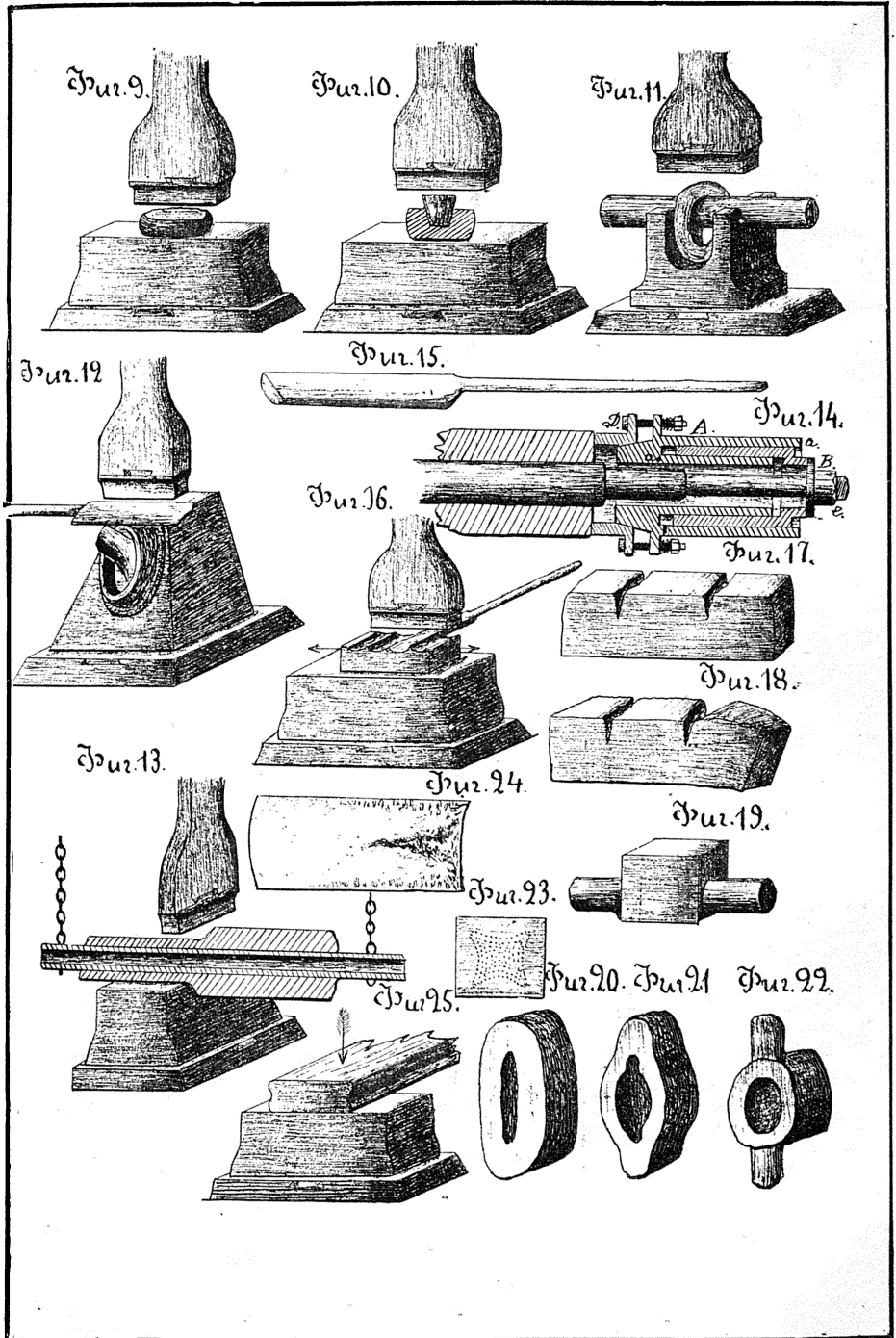
Фиг. 9. Спаянивание болванки. Фиг. 10. Пробиивание отверстия. Фиг. 11. Разводка колец. Фиг. 12. Разводка баб- дажа. Чнг. 13. Ковка на оправкѣ. Фиг. 14. Приборъ для вытягиванія оправки. Фиг. 15. Раскатка. Фиг. 16. Раскатка болванки. Фиг. 17, 18 и 19. Изготовленіе колычатого вала. Фиг. 20, 21 и 22. Изготовленіе цапфальныхъ колець. Фиг. 23. Ляній паташеій при холодной ковкѣ. Фиг. 24. Разрѣвъ болванки. Фиг. 25. Распоазаніе металла при поверхкѣ ковкѣ.
