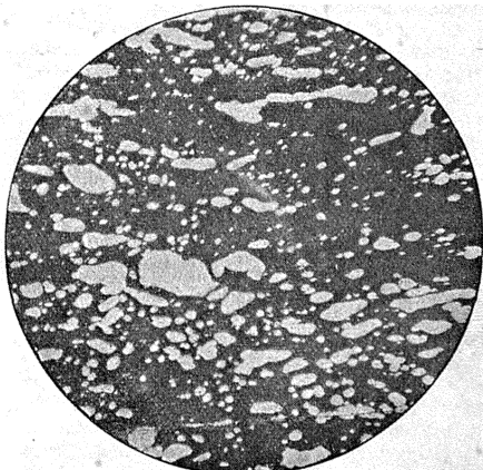
Фиг. 1, а и б. Разрѣзы кокса подъ микроскопомъ.
