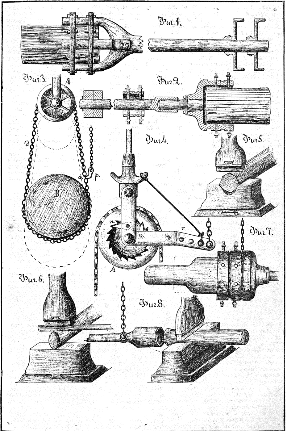
Фиг. 1 и 2. Державка при ковкѣ болванки. Фиг. 3 и 4. Приборы для поворачиванія болванки. Фиг. 5. Обжимка болванки въ 8-ми гранникъ. Фиг. 6. Губка болванки подъ молотомъ. Фиг. 7. Заготовка болванки. Фиг. 8. Осаживаніе металла.
