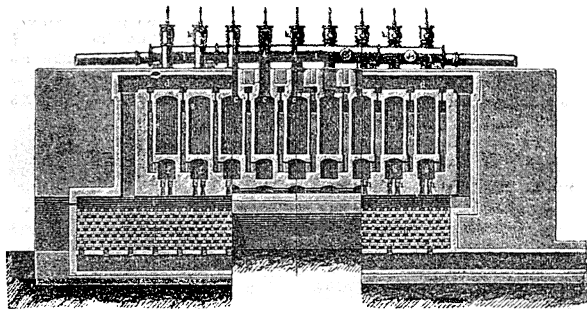
Фиг. 5. Печь Отто-Гоффмана.
